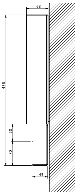
BOČNÍ POHLED
