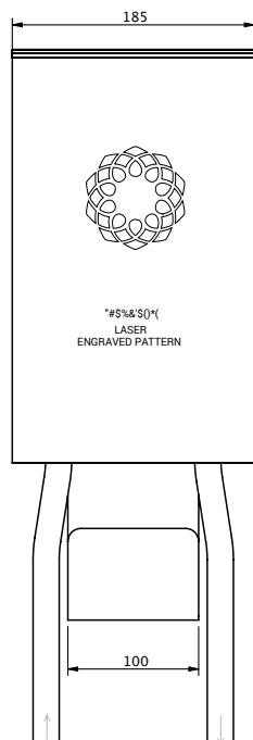
HORNÍ POHLED
